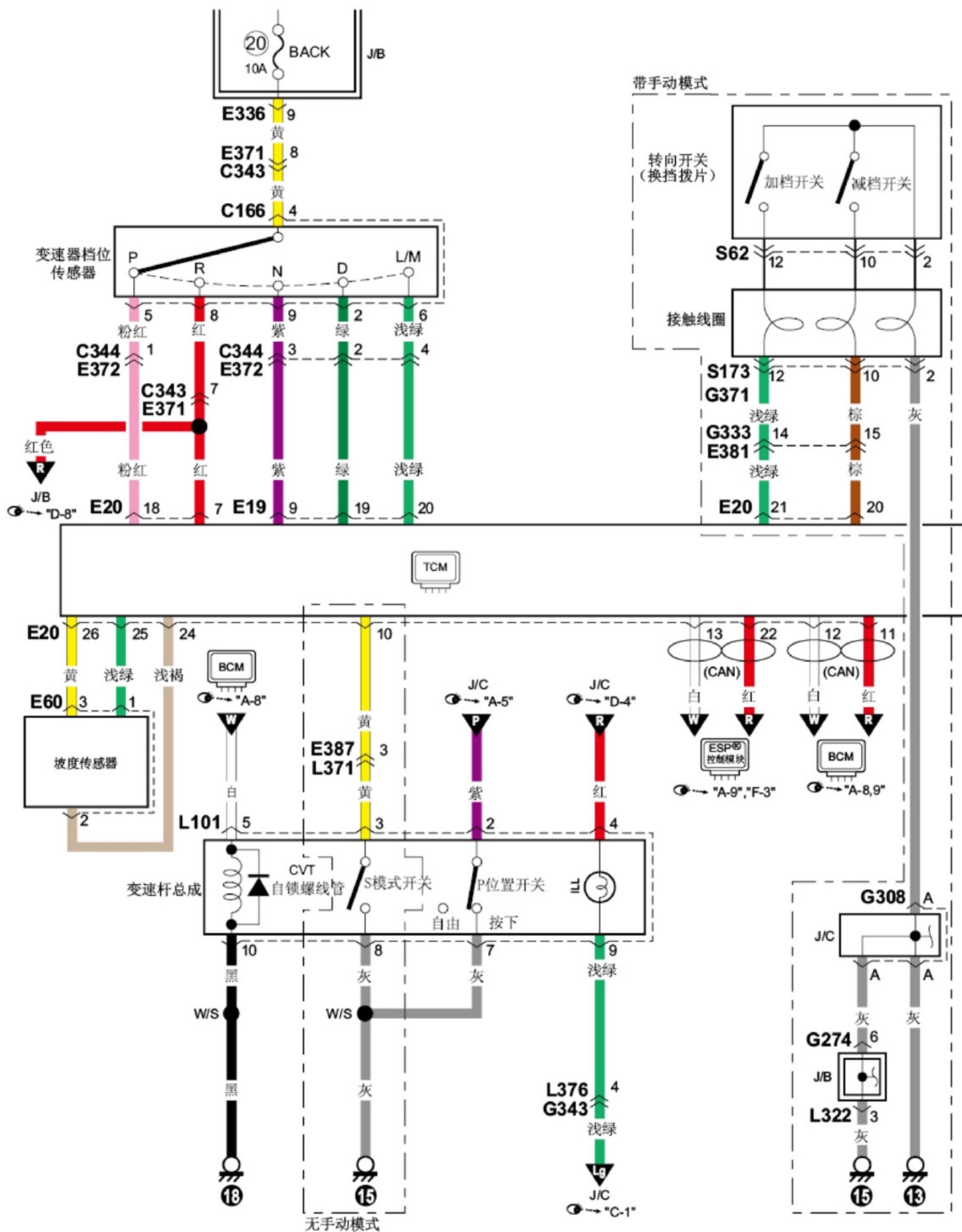
A-6 CVT控制系统电路图
